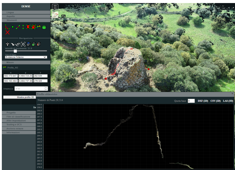
Il CloudViewer di GeoSDH per la visualizzazione, l'analisi, la misura e l'estrazione di informazioni delle nuvole di punti 3D
